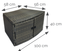
Placard avec double porte
